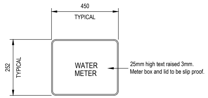
LID DETAIL
